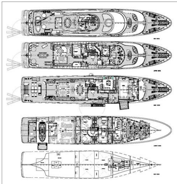
Deckplans
